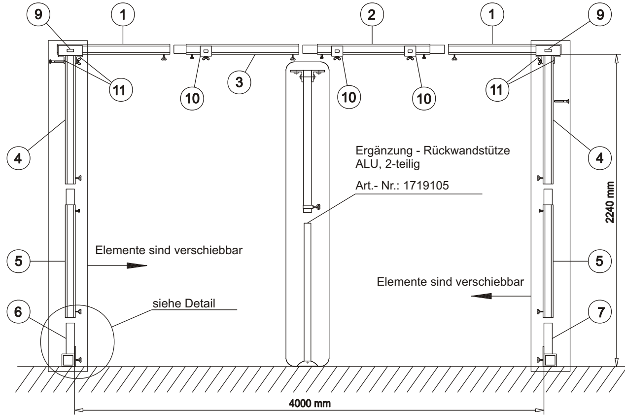
Alu - Profil 0437
